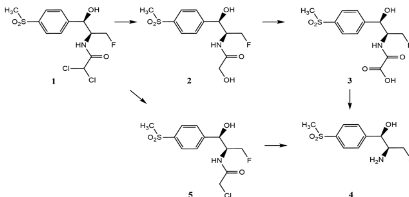
Рисунок 1. Схема метаболизма флорфеникола
